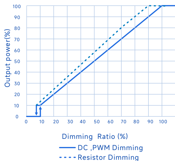
输出功率Vs.调光信号(B机型)
